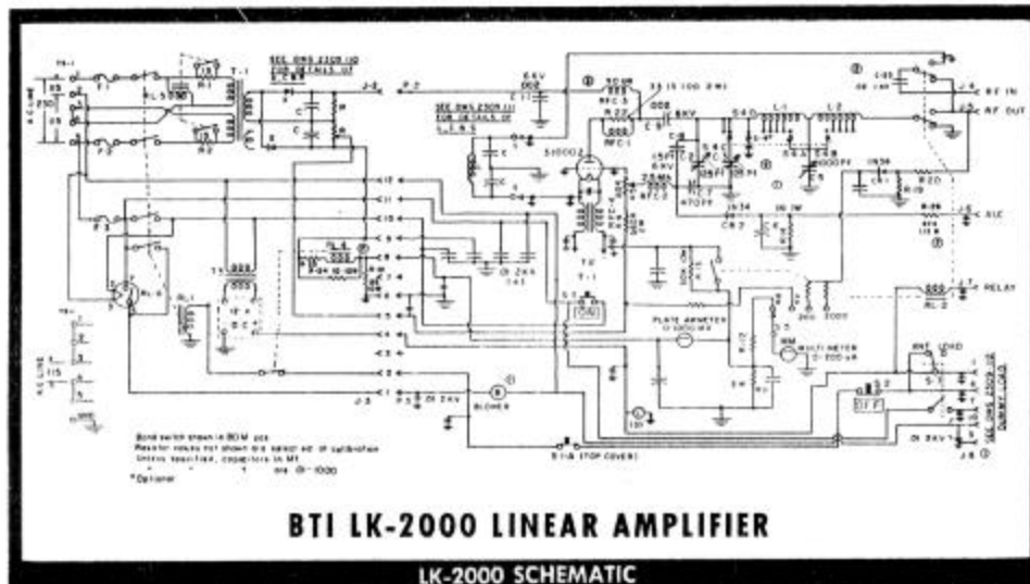
LK-2000 SCHEMATIC
